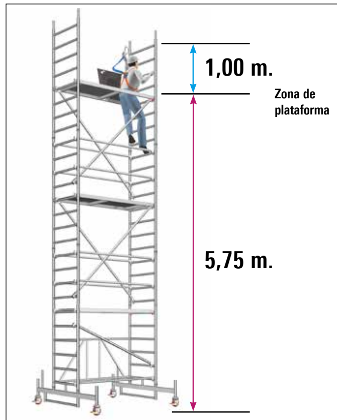
Fig. 2: Alturas mínimas para el uso del EPI
