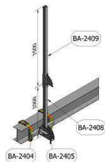
BARANA METÀL·LICA DE SEGURETAT
