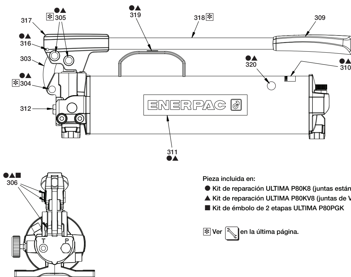
Fig. 1 Palanca, mango y etiquetas
