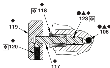
SECCIÓN C - C
