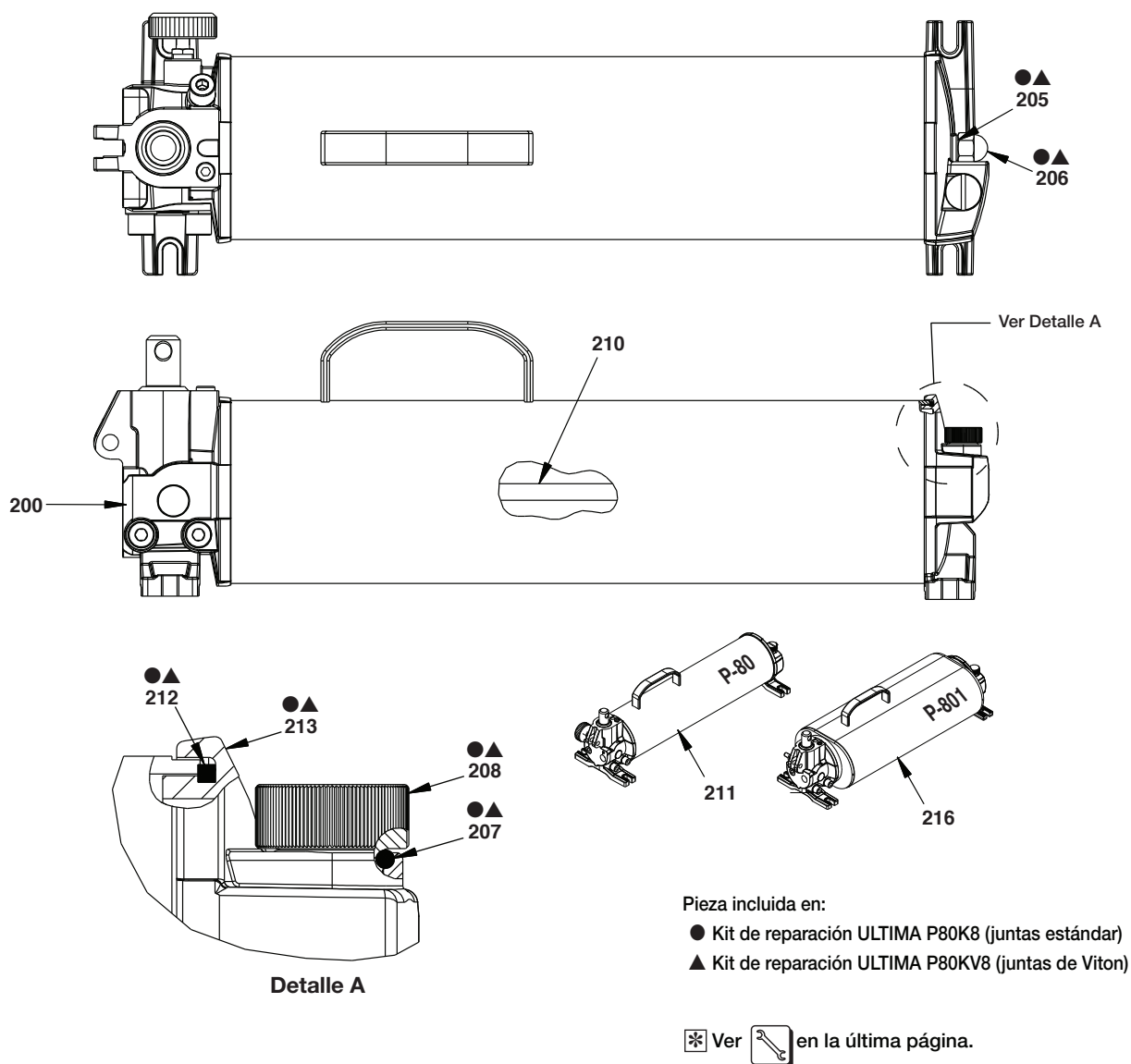
Fig. 2 Depósito de la bomba
