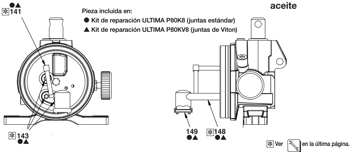
Lista de repuestos, Fig. 8
