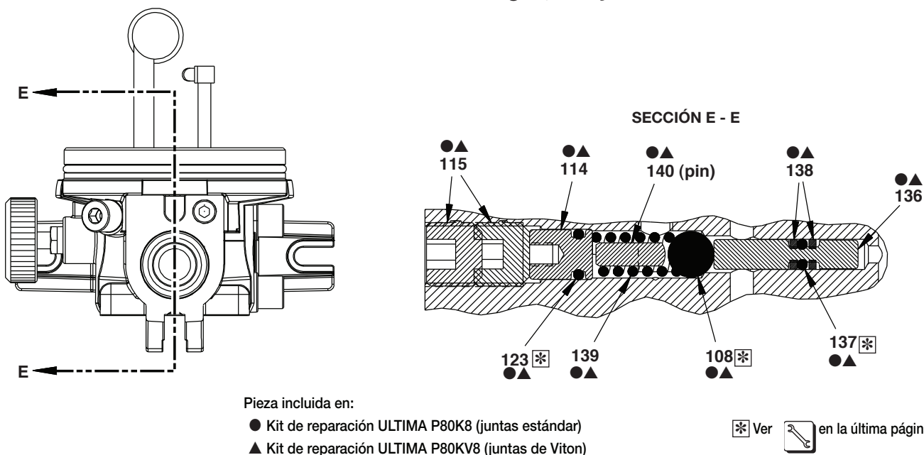
Fig. 7, Conjunto de válvula de derivación
