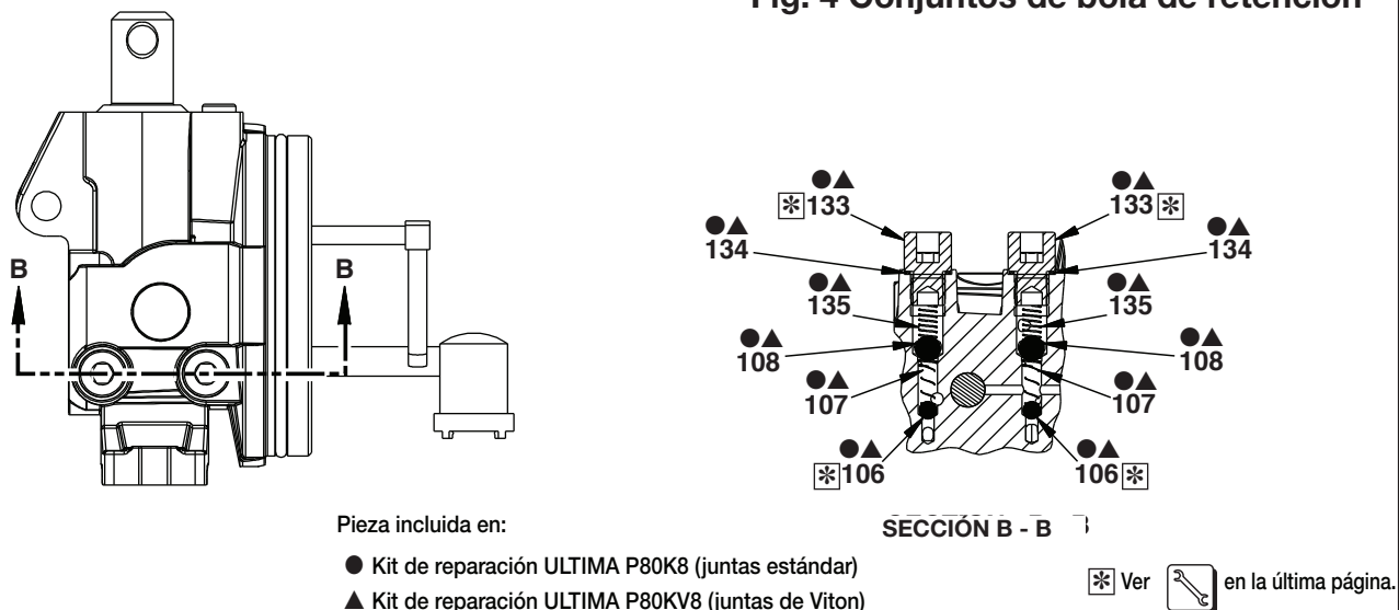
Fig. 4 Conjuntos de bola de retención
