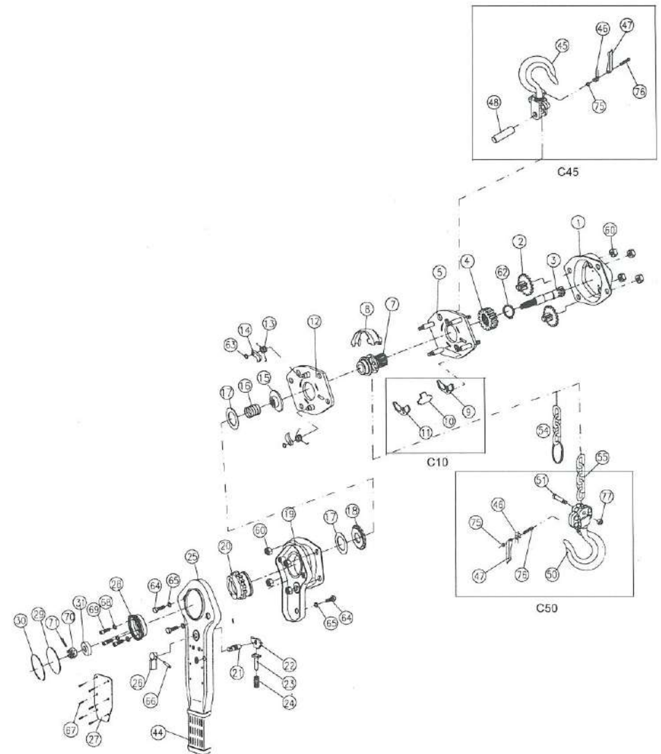
DESPICCE DE POLIPASTO 0,5 - 9TN.
